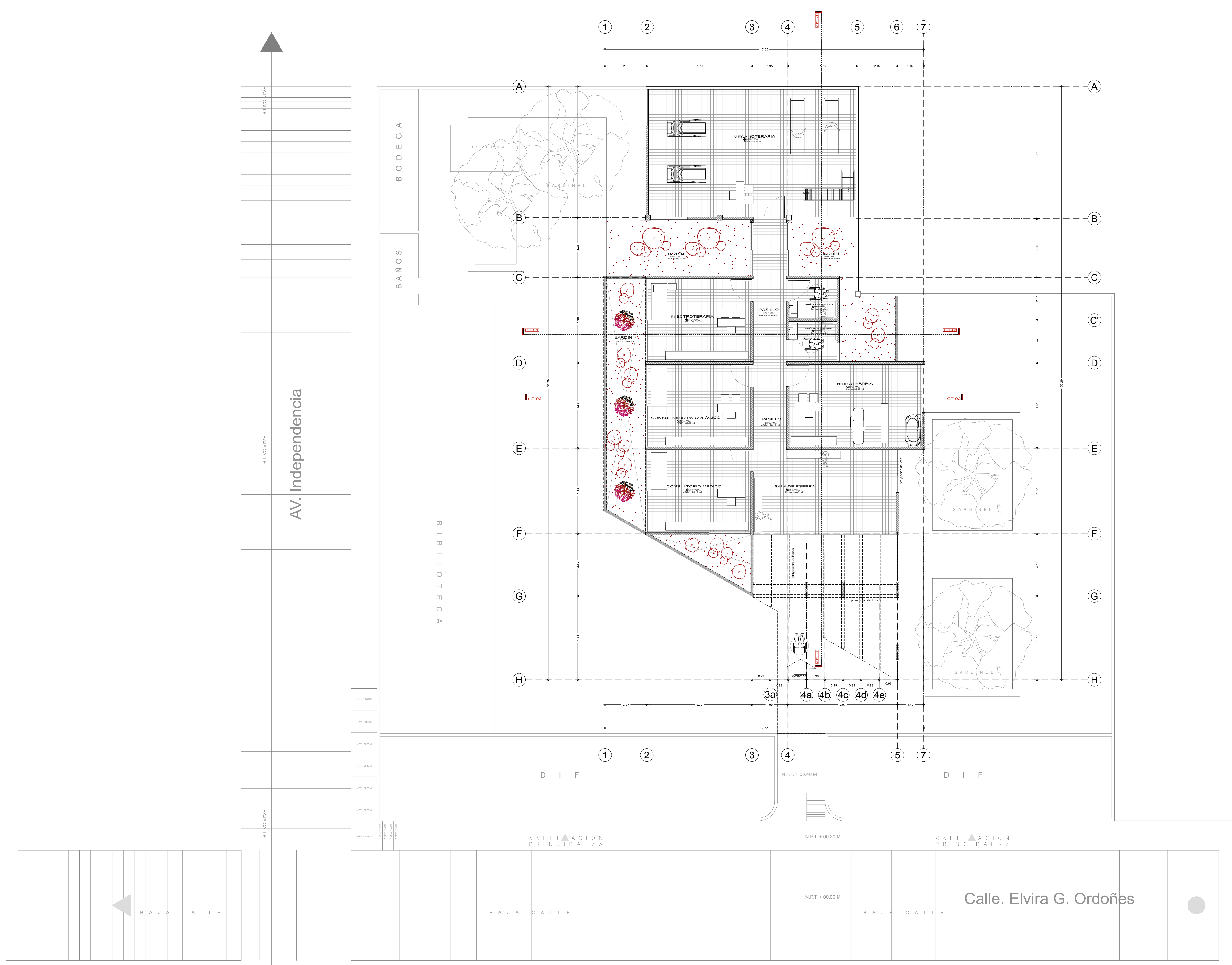
PLANTA DE ARQUITECTÓNICA ESCALA: 1:100 ESCALA GRÁFICA
